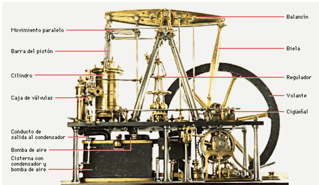
Máquina de vapor
